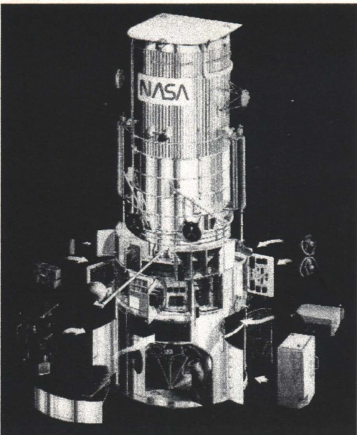
Das HST in seinen Baugruppen
